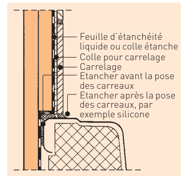
Détail 31 : Raccordement à une paroi FERMACELL simple couche avec doublage au-dessus du bac de douche ou de baignoire.
