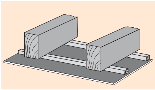
Détail 9 : Parement fixé sur lattage porteur
