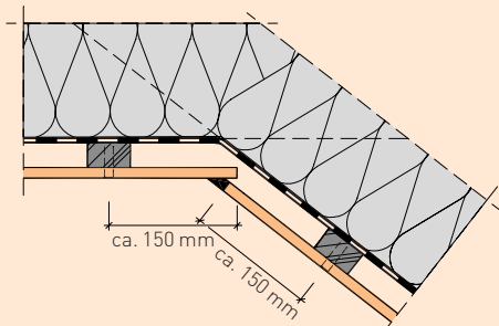
Détail 21 : Pan de toiture – plafond
