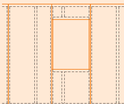
Détail 6 : Ouverture de fenêtre avec joint de parement vertical sans décalage
