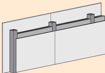
Détail 1 : Joints des plaques dans le cas d'un parement monocouche
