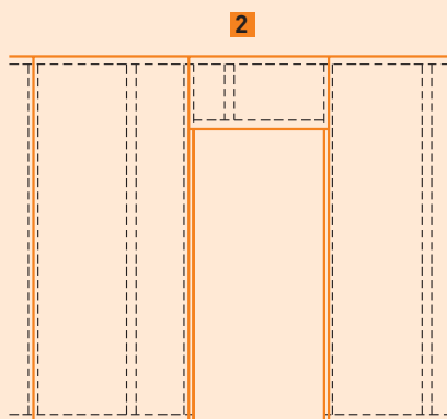
Détail 5 : Ouverture de porte avec joint de parement vertical sans décalage
