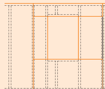
Détail 8 : Ouverture de fenêtre avec joint de parement horizontal
