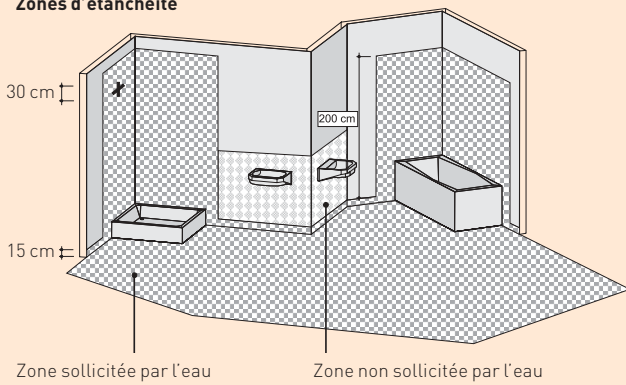
Figure 27 : Surfaces sollicitées par l'eau
