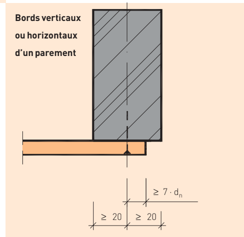
Détail 13 : Ecartement sur un montant périphérique
