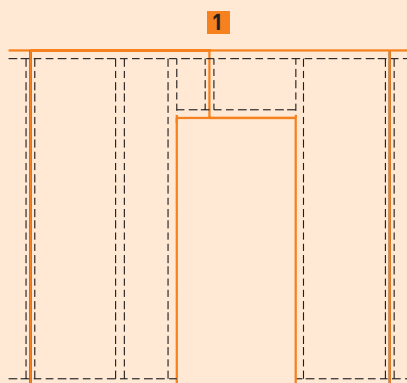
Détail 3 : Ouverture de porte avec décalage du joint
