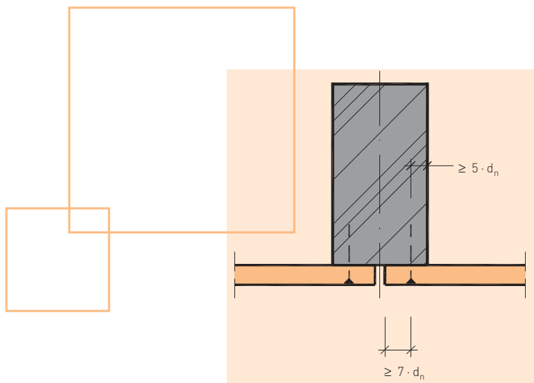
Détail 12 : Ecartement sur un montant intermédiaire
