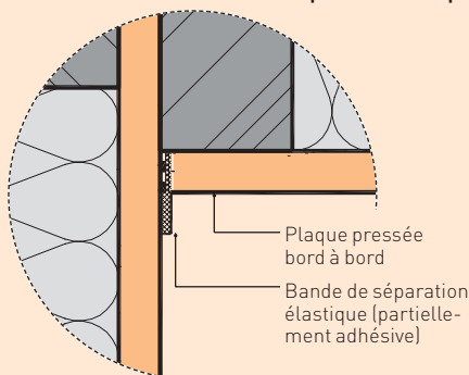
Détail 27 : Joint bord à bord avec bande de séparation élastique
