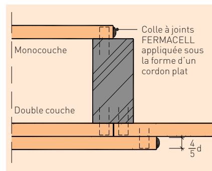
Détail 14 : Application de la colle à joints FERMACELL sur le chant vertical de la plaque à l'aide d'une cartouche de colle
