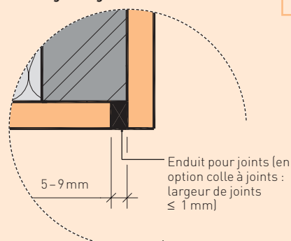
Détail 28 : Enduisage d'angles saillants
