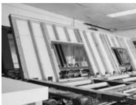
Figure 3 : Table de retournement
