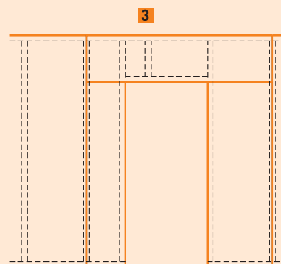
Détail 7 : Ouverture de porte avec joint de parement horizontal
