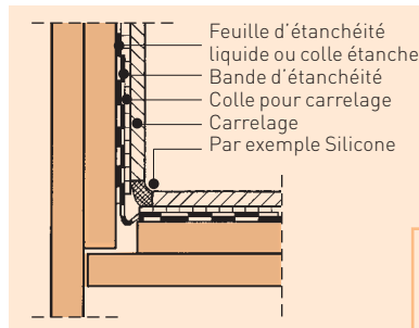
Détail 29 : Exécution d'un angle de parois dans une zone sollicité par l'eau
