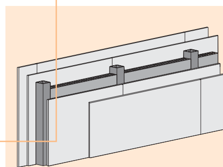
Détail 2 : Joints des plaques dans le cas d'un parement bicouche
